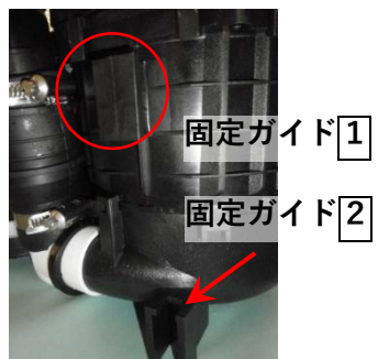
② 固定ガイド1に防振ゴムが付いている場合は取り除きます。
