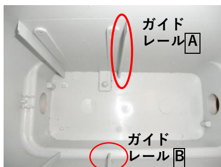
① 旧本体ケース (2011 年以前のモデル)
