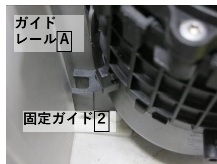
③ 本体ケースの底部の突起に固定ガイド2を乗せます。
