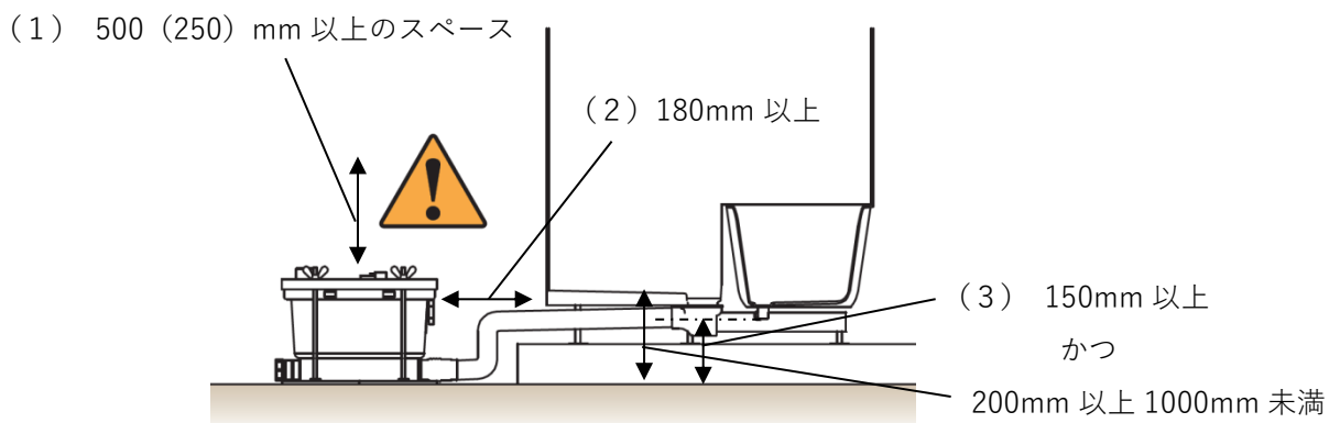
図1 設置に必要な寸法
